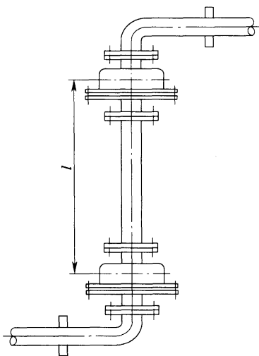
图 7.11.5-2 球形补偿器球心距的安装长度
