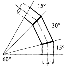
(b) 60° 斜接弯头
