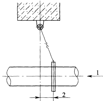
图 7.12.3 有热位移管道吊架安装 1—管子膨胀方向;2—1/2 位移值
