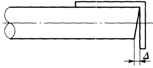
图 5.2.4 管子切口端面倾斜偏差
