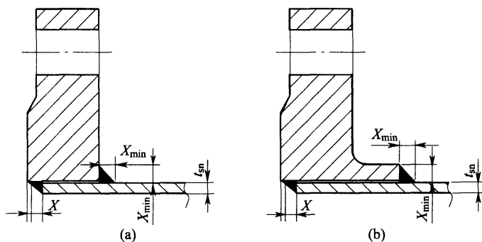
图 6.0.7-1 平焊法兰与管子的连接
