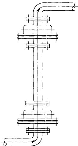
图 7.11.5-3 球形补偿器的安装方向
