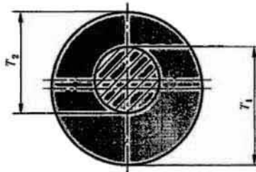
图 1 焊条偏心度测量示意图
