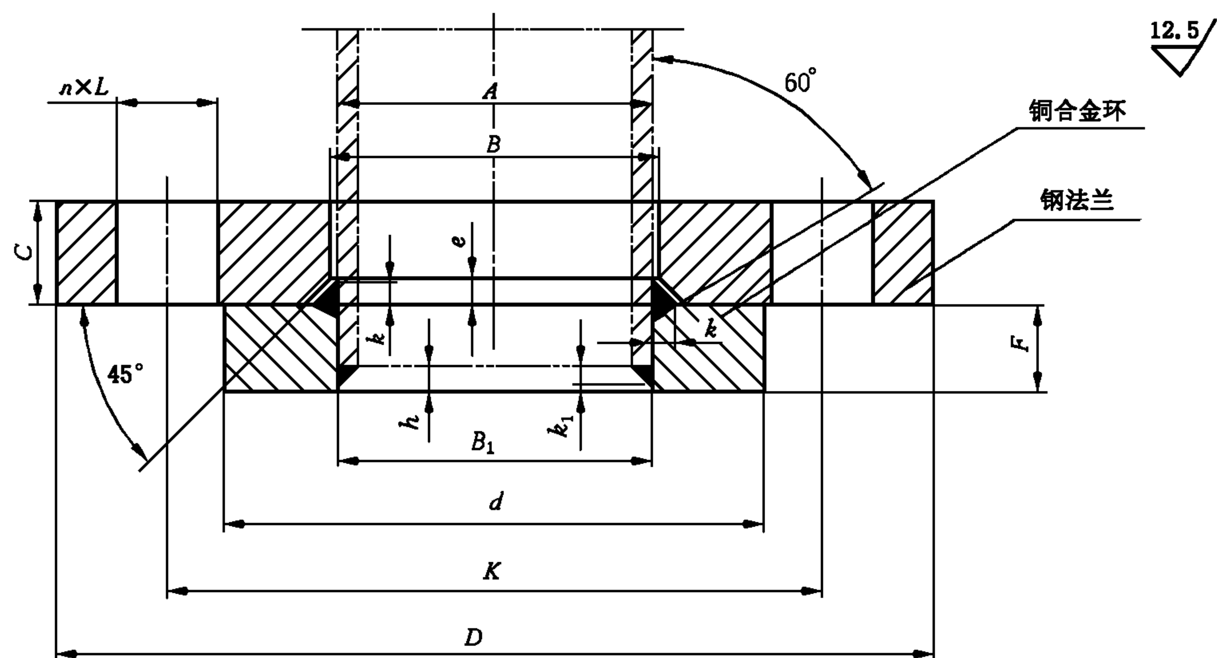
图 1 铜合金平焊环松套钢法兰
