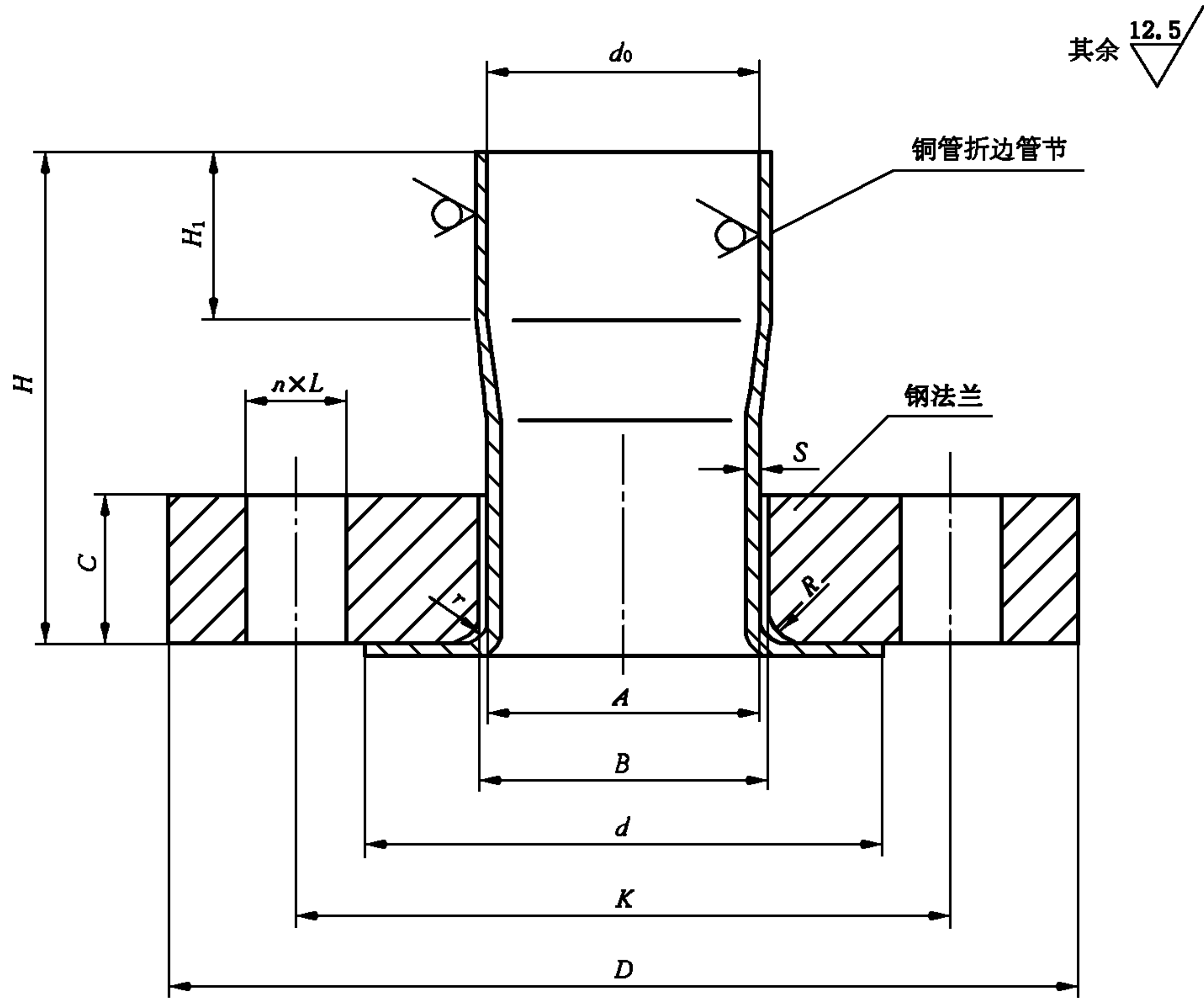
图 1 铜管折边松套钢法兰(A 型)
