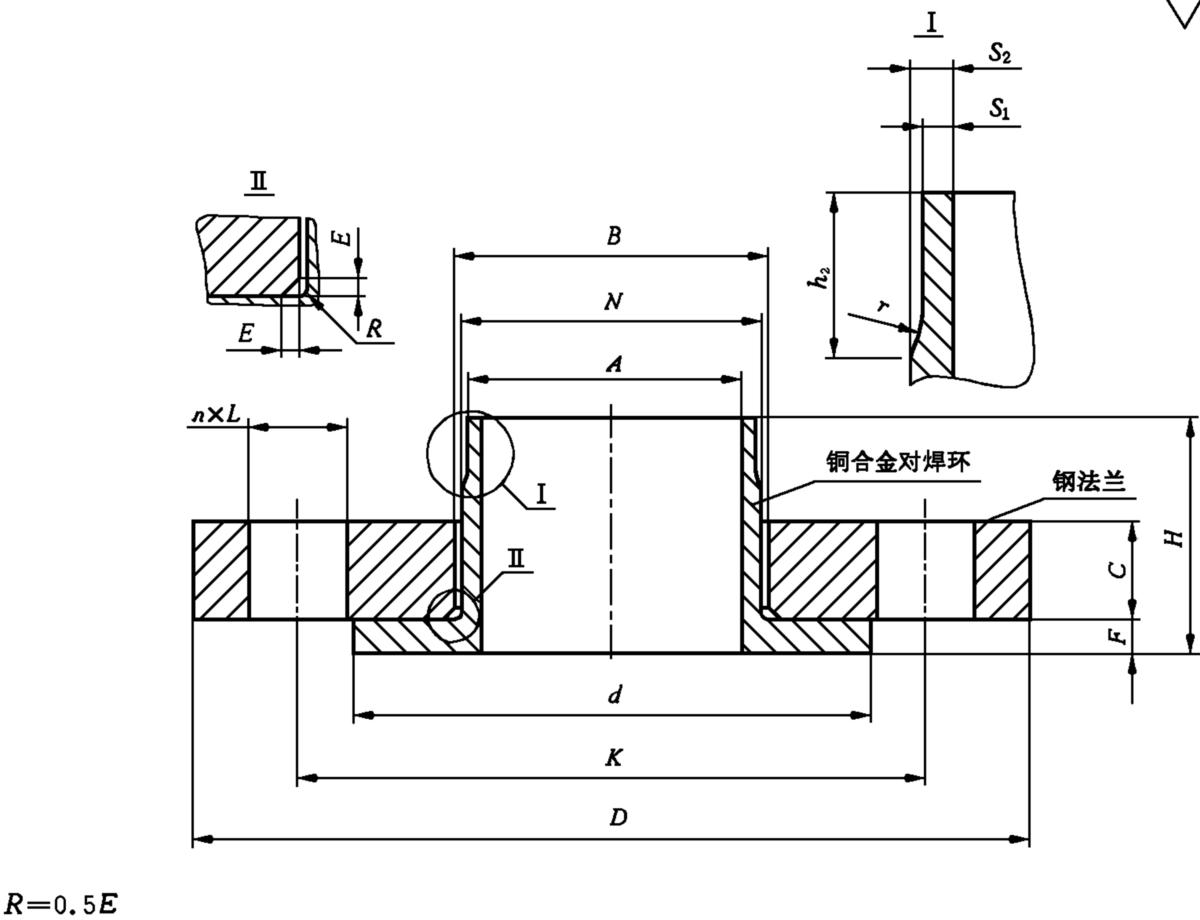
图 2 铜合金对焊环松套钢法兰(B型) 表 5 PN6 铜合金对焊环松套钢法兰尺寸
