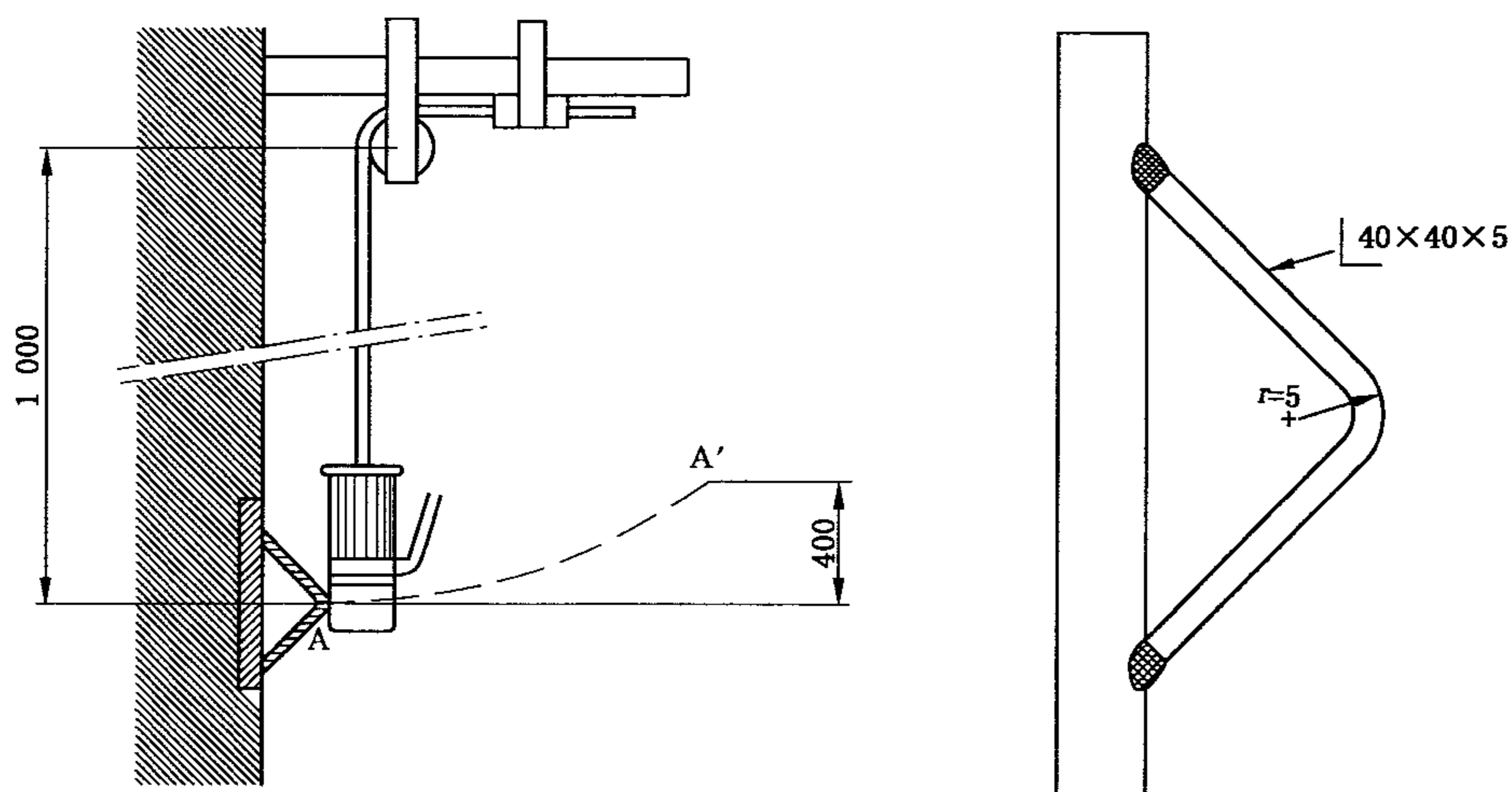
图 3 摆动冲击试验装置
