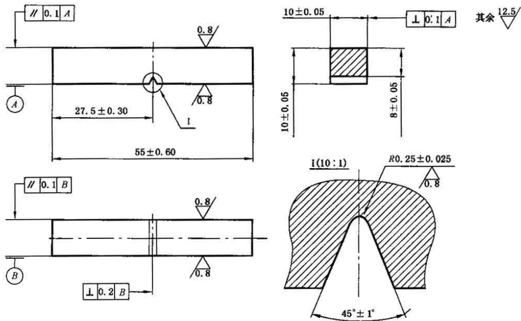
图3 夏比V型缺口冲击试样
