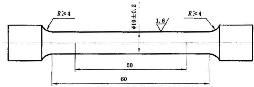
图2 熔敷金属拉伸试样
