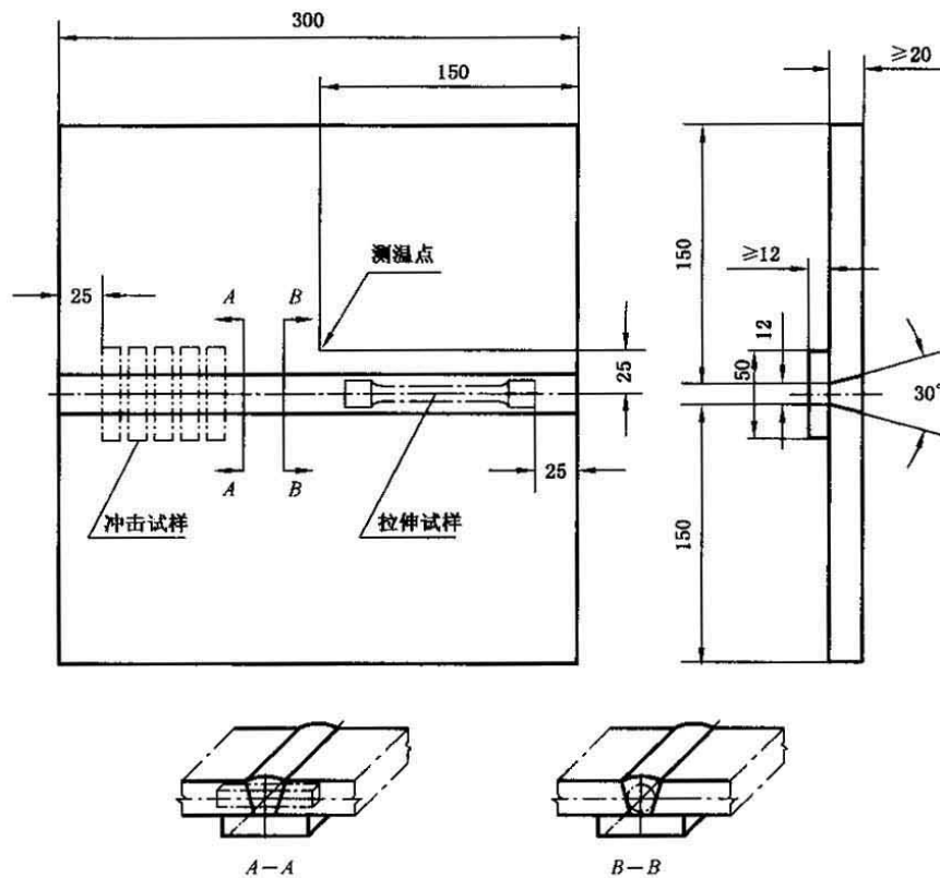
图 1 射线探伤和力学性能试验的试件制备
