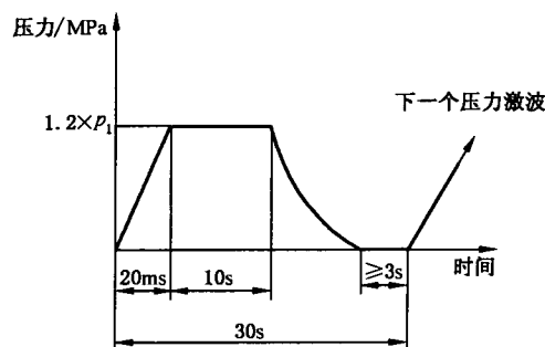
图 3 试验间隔
